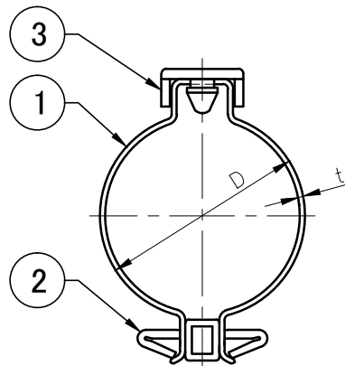
A矢视图
