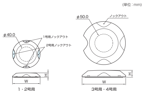
寸法表
