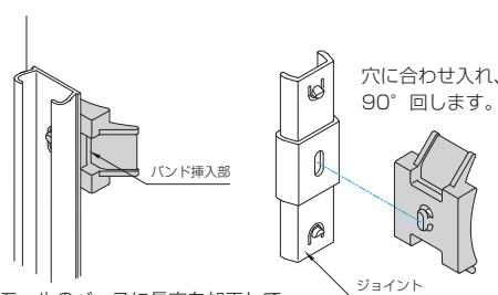
モールのベースに長穴を加工して固定ベースを取付けます。またジョイントの長穴に合わせ入れ、固定ベースを取付けることもできます。
