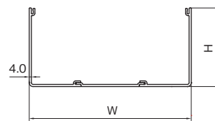
300×100型・300×150型
