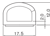
原寸大断面図 (単位：mm)
