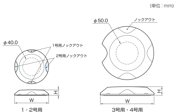
寸法表
